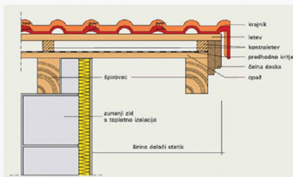
VZDOLŽNI PREREZ DETAJLA ZAKLJUČKA STREHE
